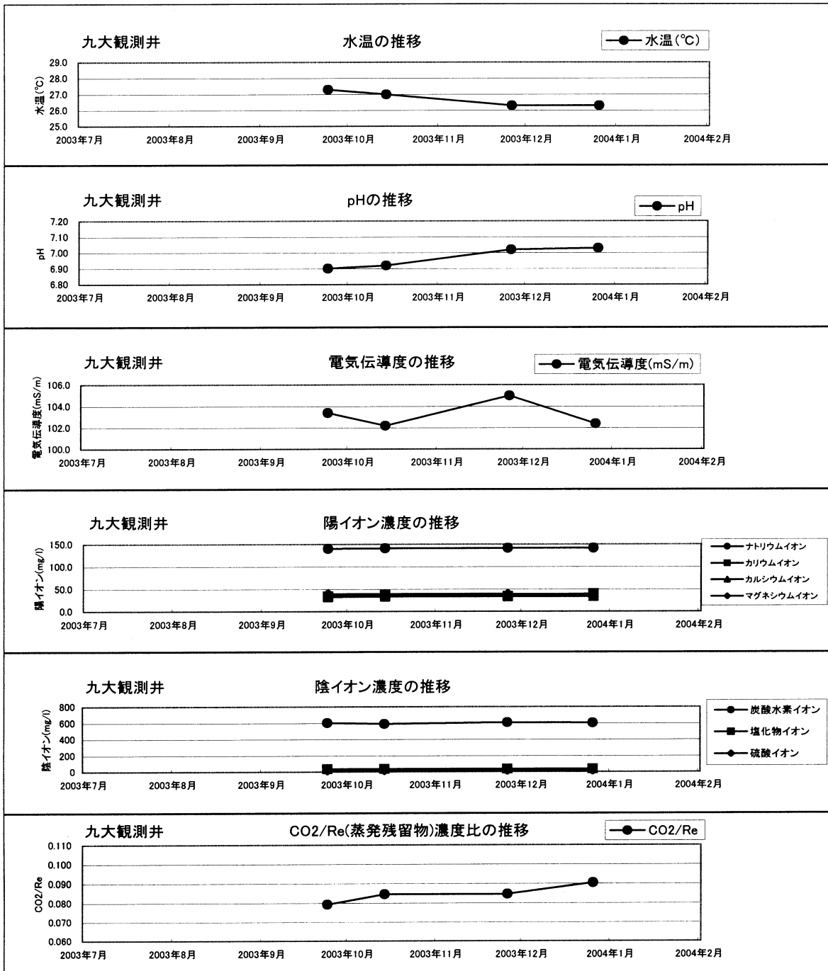
九大島原温泉観測井の温度・pH・電気伝導度・主要化学成分濃度・CO 2 /Re(蒸発残留物)濃度比の推移
