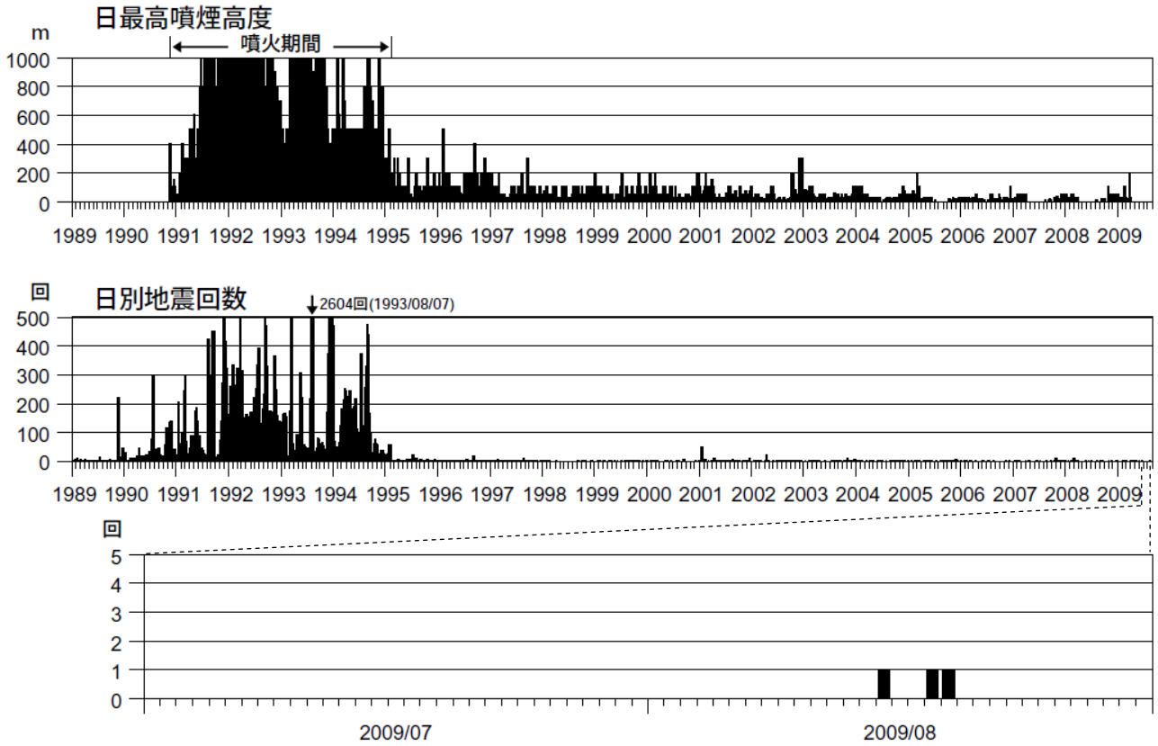
図 2 雲仙岳 火山活動経過図（1989 年 1 月～2009 年 8 月） 1995 年 2 月の噴火活動停止以降、噴煙活動、地震活動ともに静穏な状態で経過しています。
