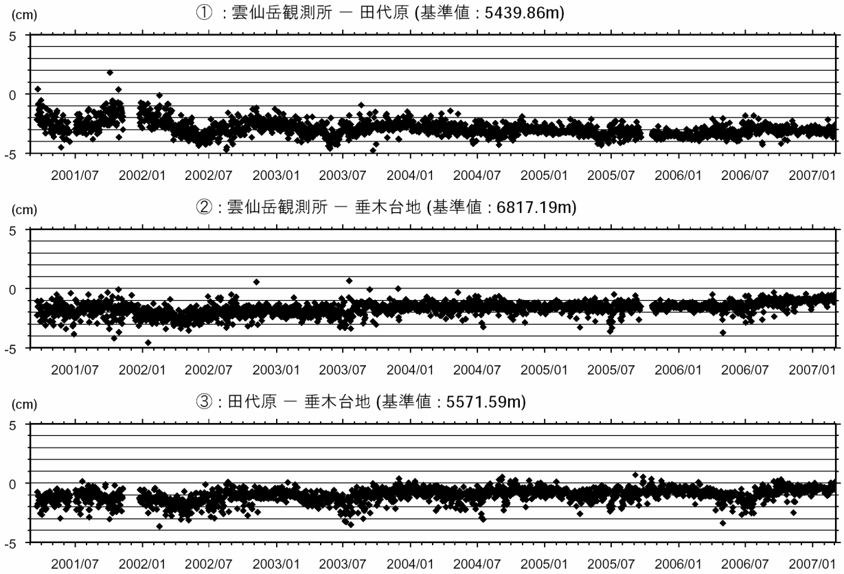
図3 雲仙岳 GPSによる基線長変化(2001年3月20日~2007年2月28日) 火山活動に起因するとみられる変化は認められませんでした。
