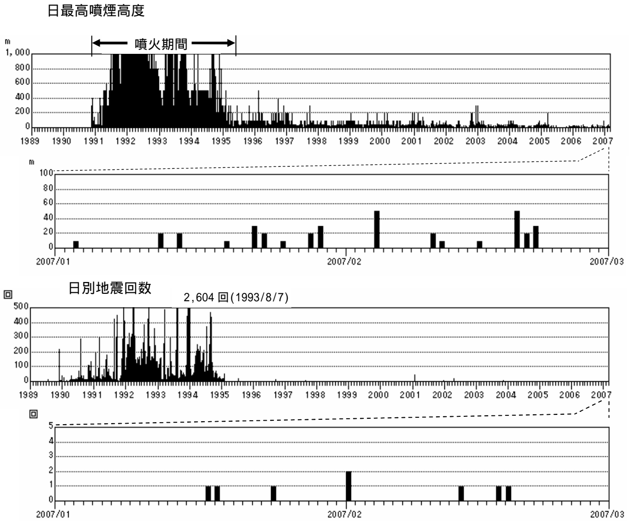
図2 雲仙岳 火山活動経過図(1989年1月~2007年2月)
