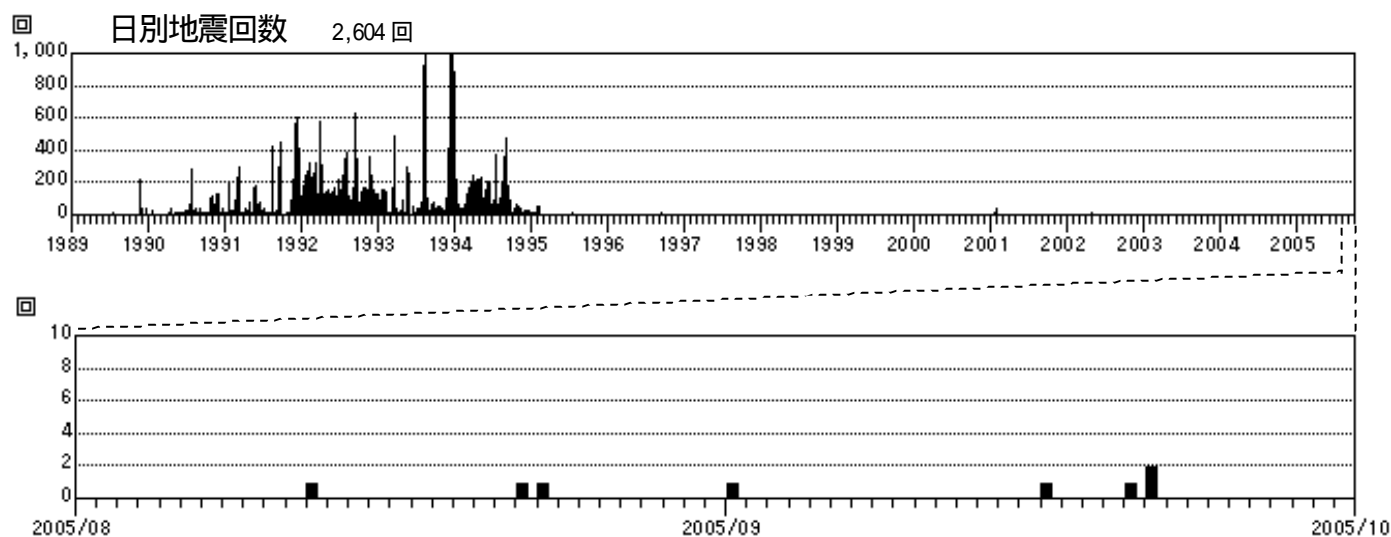
図2 地震活動経過図
