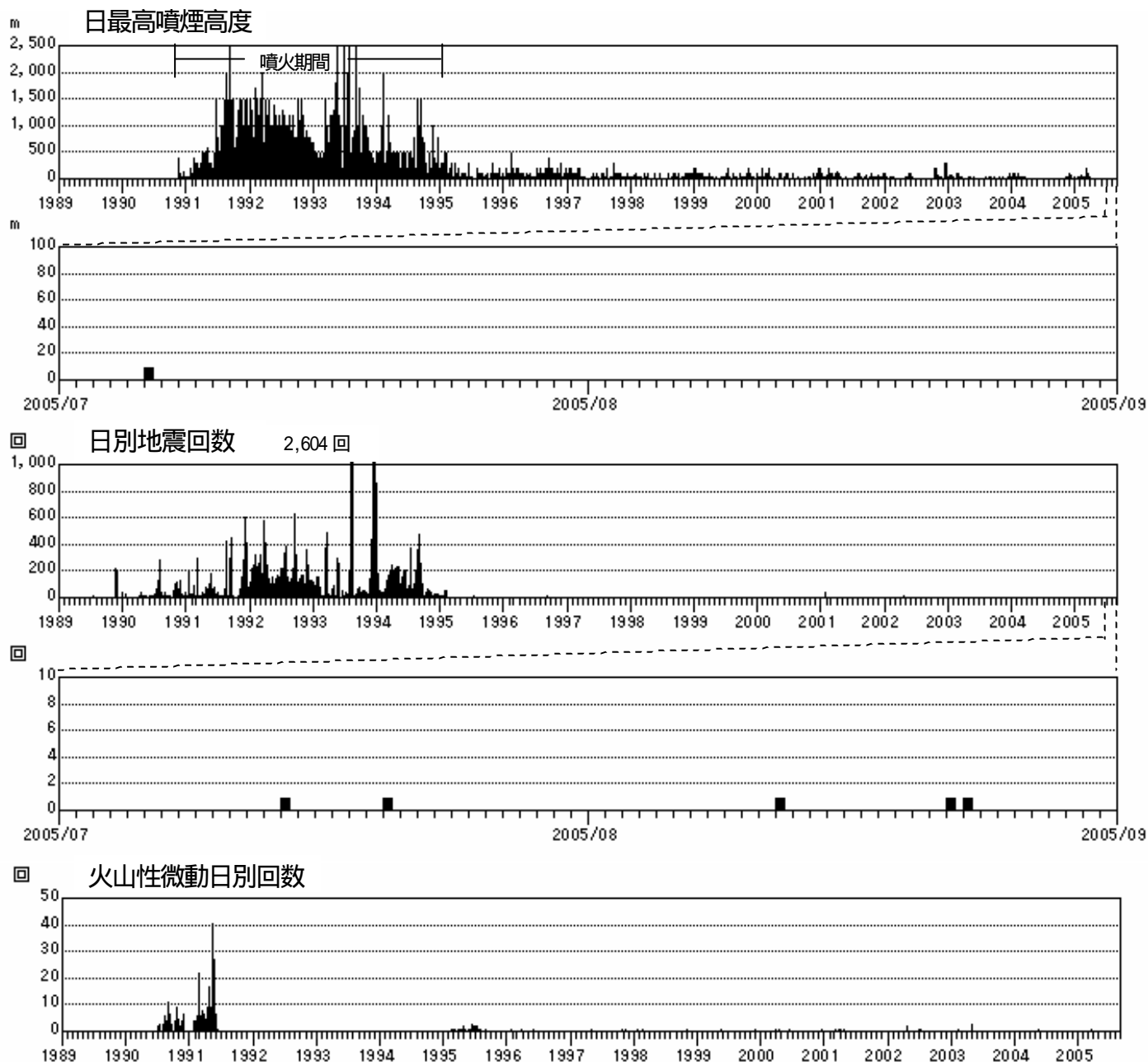
図1 火山活動経過図(1989年1月1日～2005年8月31日)
