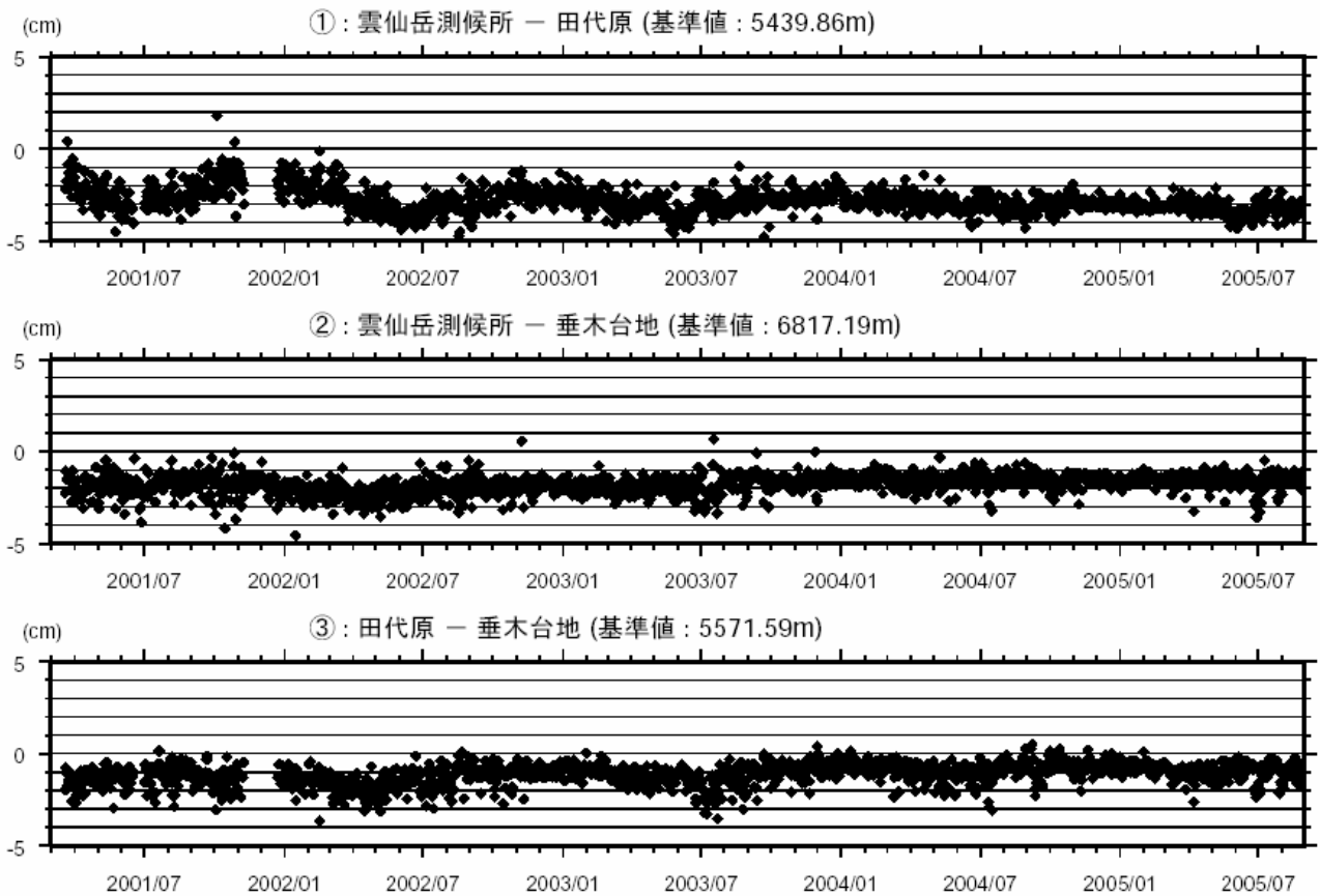
図2 GPSによる基線長変化(2001年3月20日~2005年8月31日) 火山活動に起因する変化はありませんでした。
