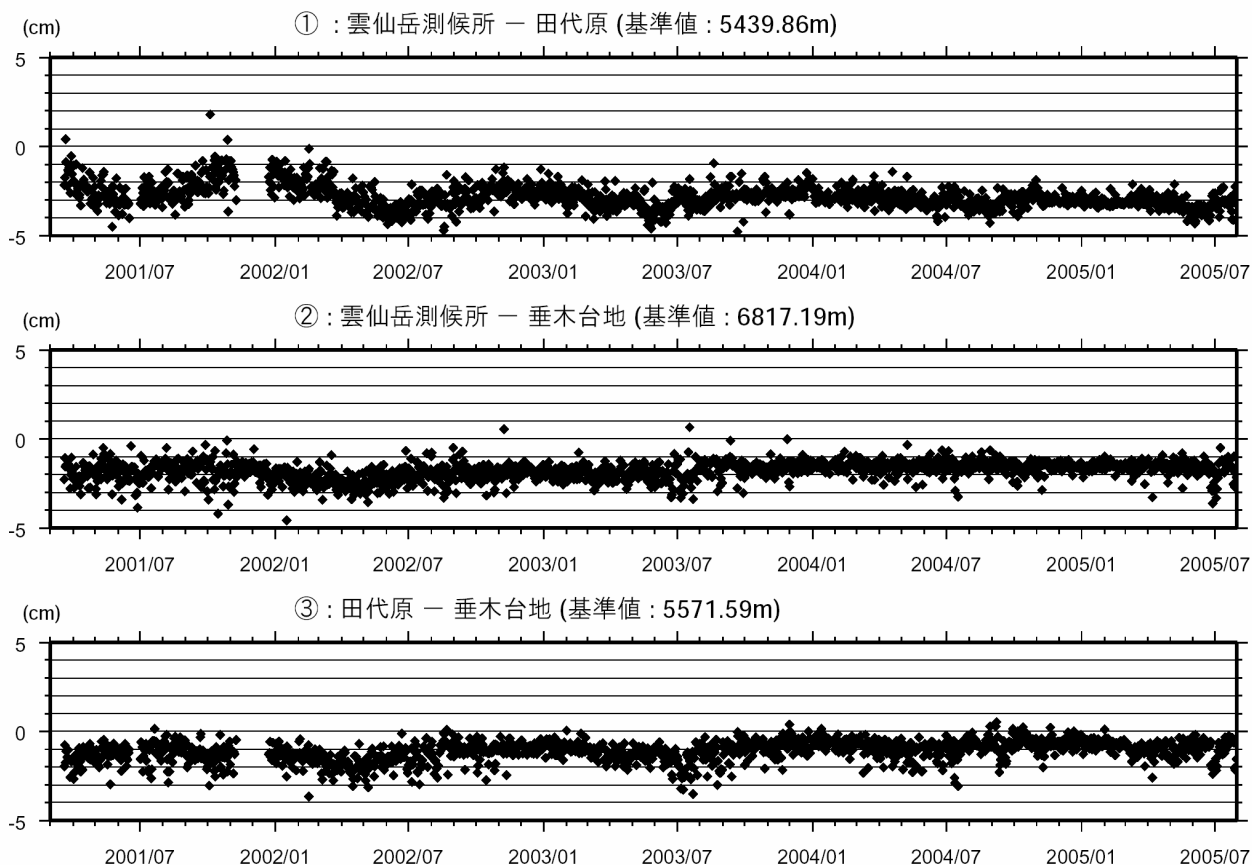
図2 GPSによる基線長変化(2001年3月20日~2005年7月31日) 火山活動に起因する変化はありませんでした。
