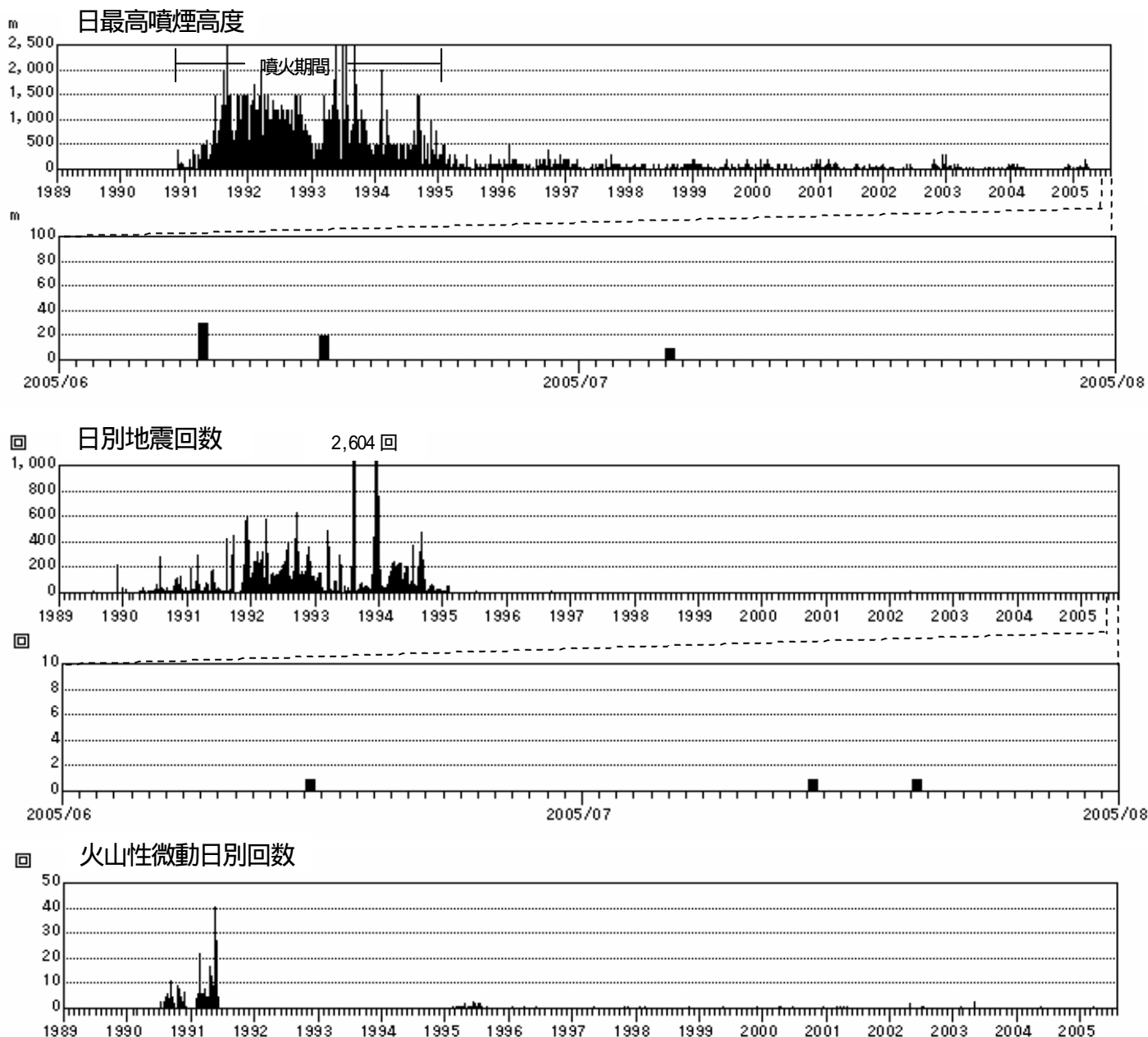
図1 火山活動経過図(1989年1月1日～2005年7月31日)
