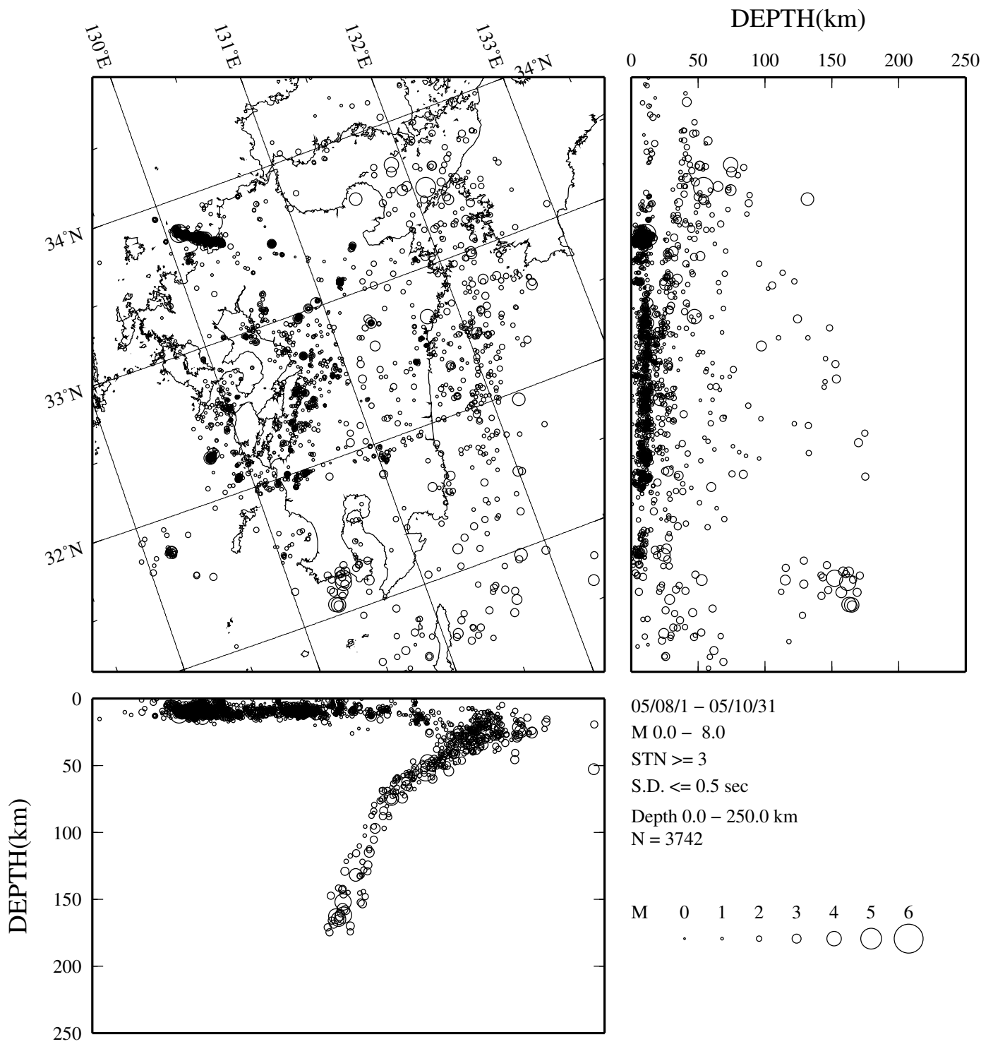
震源分布 (2005年8月~2005年10月)
