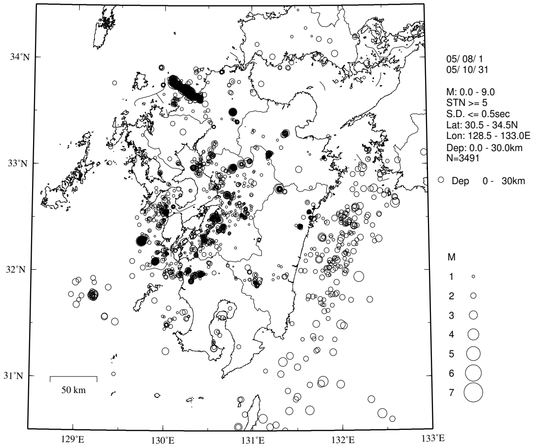
震央分布 (深さ \leq 30 Km)
