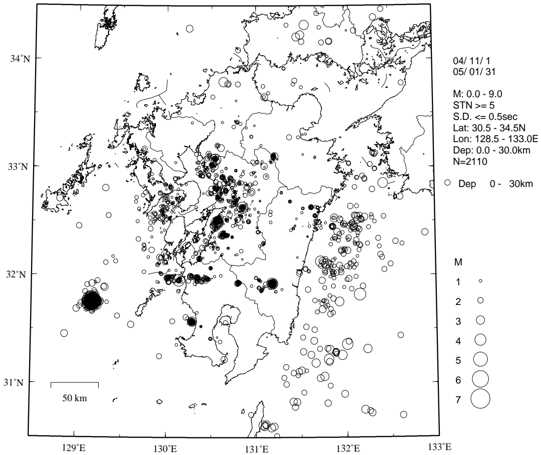
震央分布 ( 深さ 30 Km )
