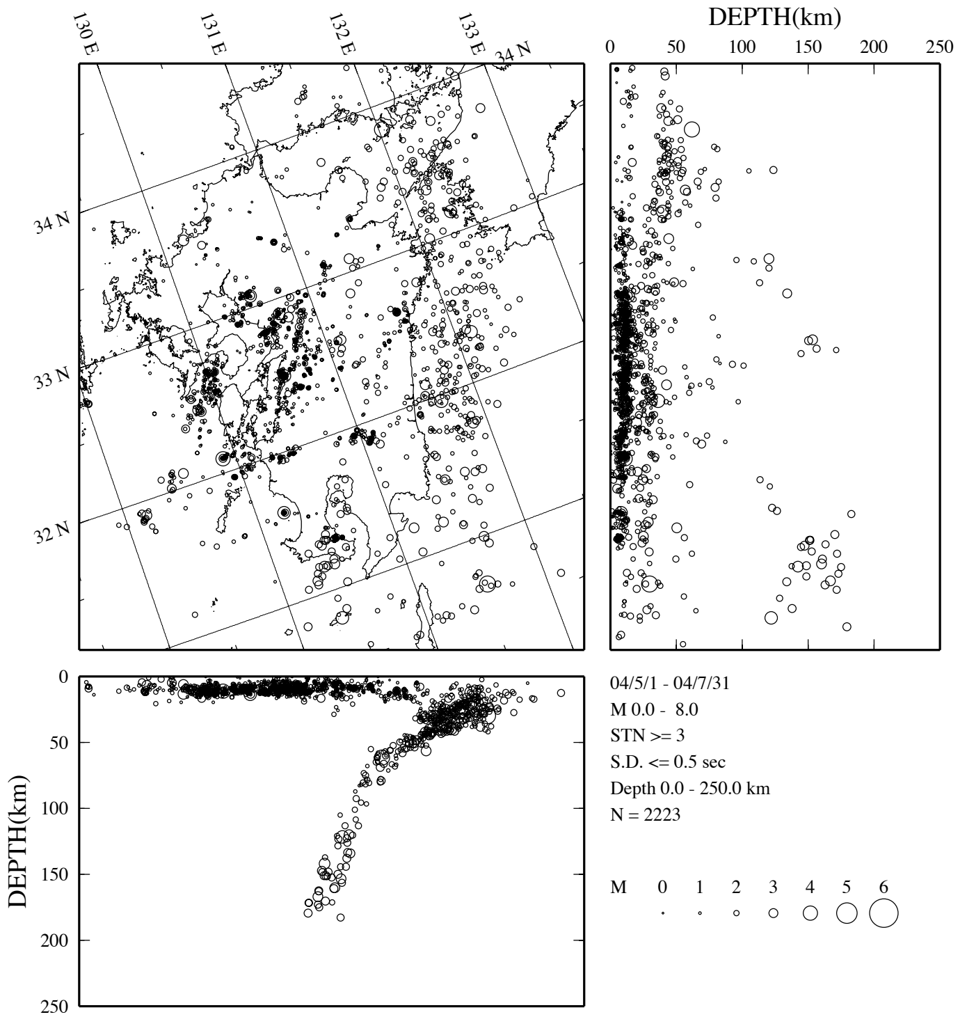
震源分布 ( 2004年5月 ~ 2004年7月 )
