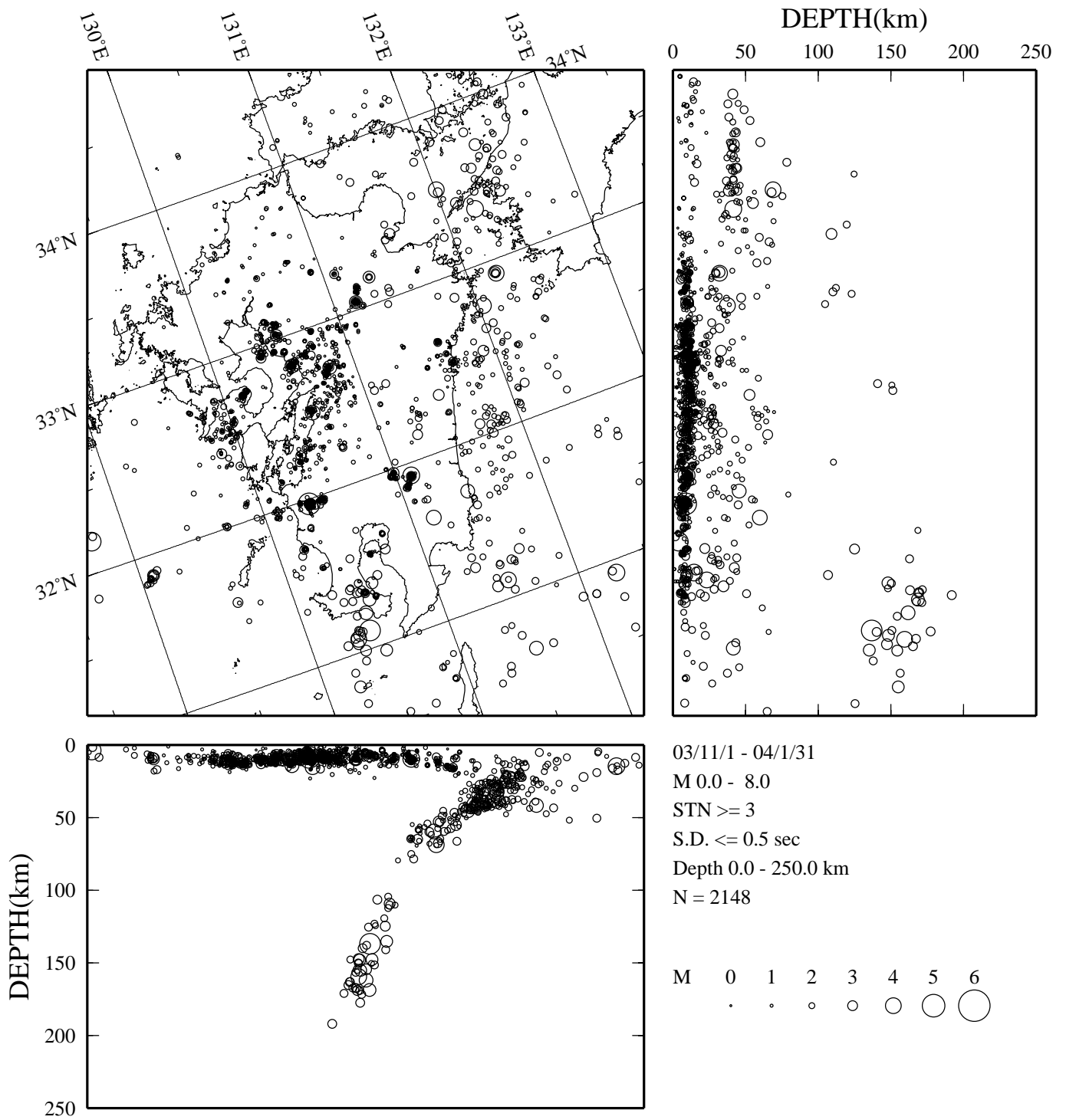
震源分布 ( 2003年11月 ~ 2004年1月 )
