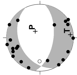
03/07/12 16:45 M3.1 熊本市
