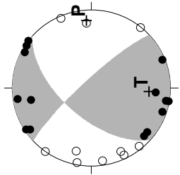
03/07/08 17:30 M3.6 八代海
