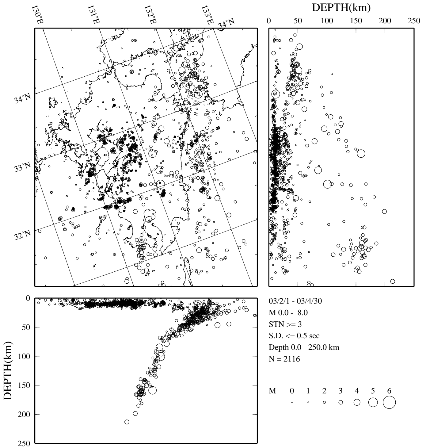
震源分布 (2003年2月~2003年4月)
