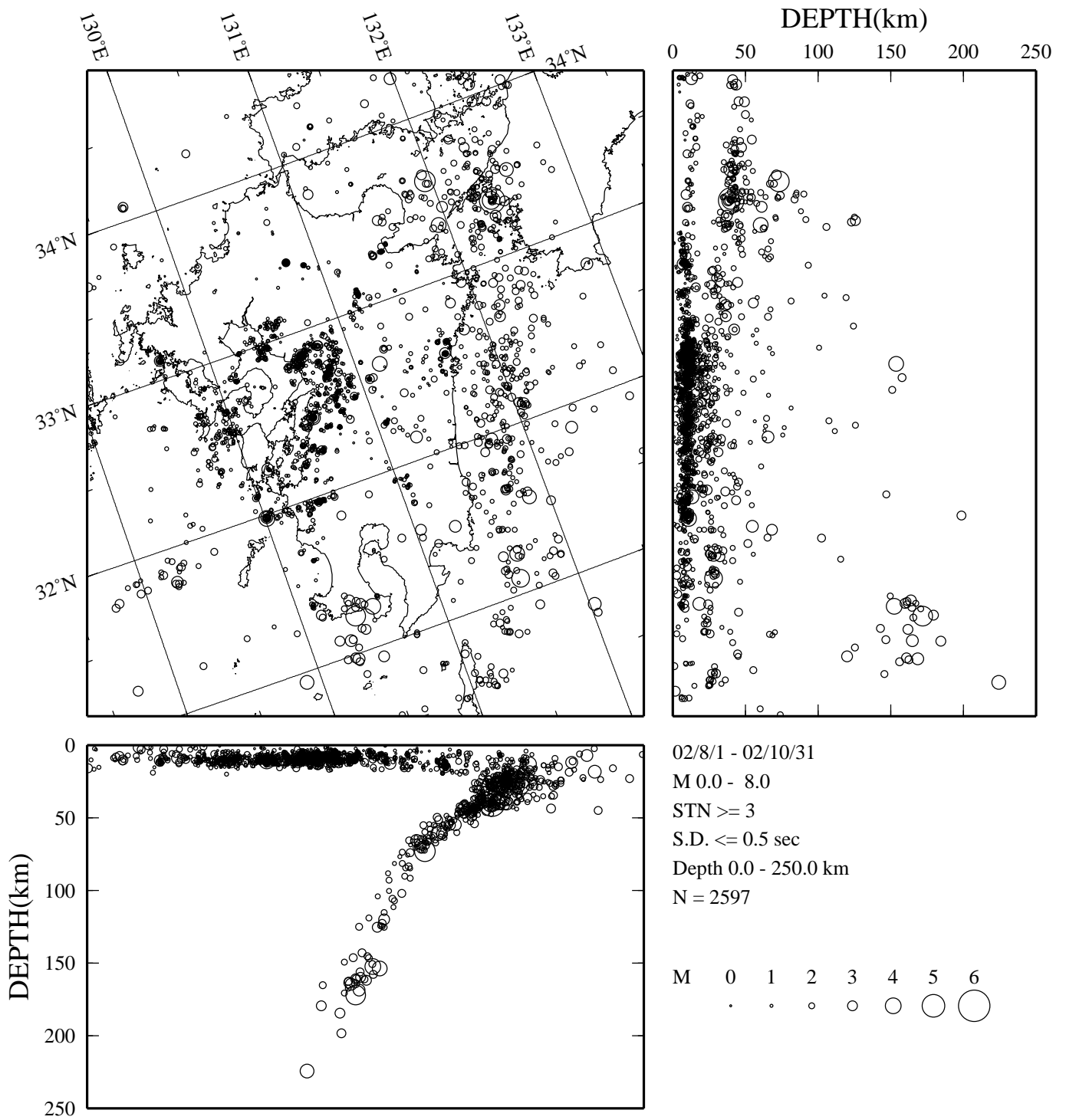
震源分布 (2002年8月~2002年10月)
