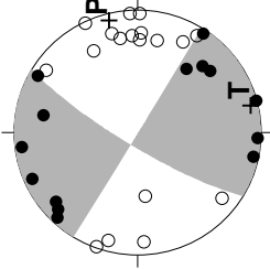
発震機構
