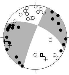
00/12/07 20:03 M4.0 天草南方
