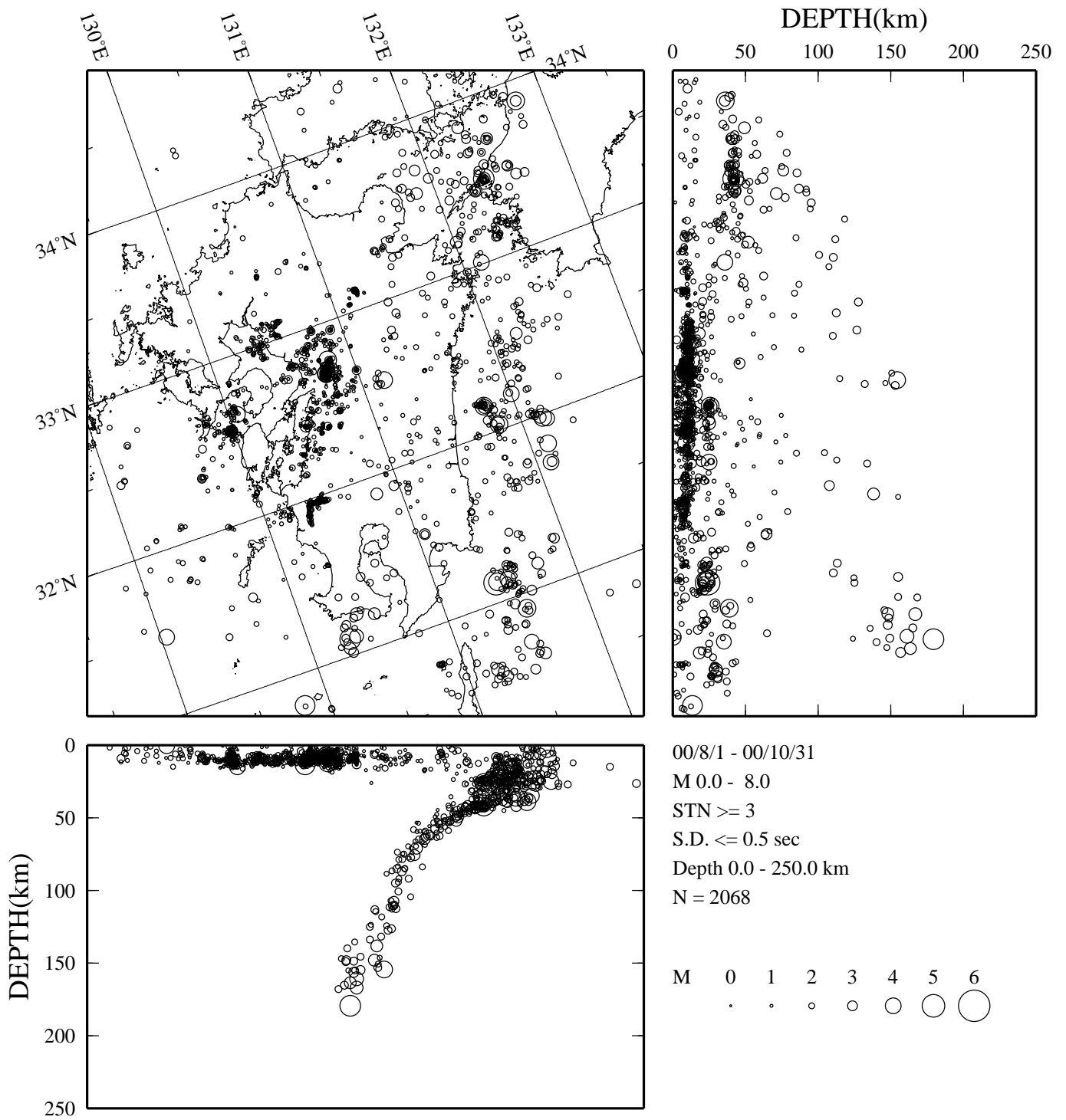
震源分布 (2000年8月~2000年10月)
