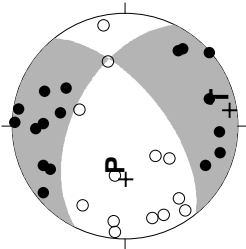
発震機構
