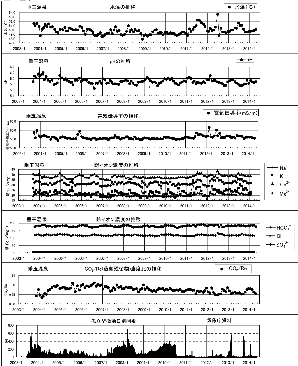
阿蘇垂玉温泉山口旅館(本湯)の水温・pH・電気伝導率・主要化学成分濃度・CO 2 /Re(蒸発残留物)濃度比の推移 (孤立型微動日別回数は気象庁資料 2003年7月～). 源泉は、中岳火口から南西約5kmに位置している。
